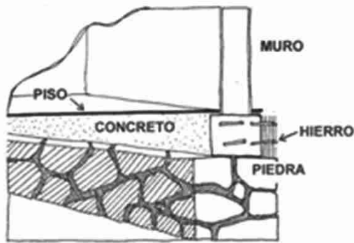
CICLOPEO CON VIGA DE AMARRE
